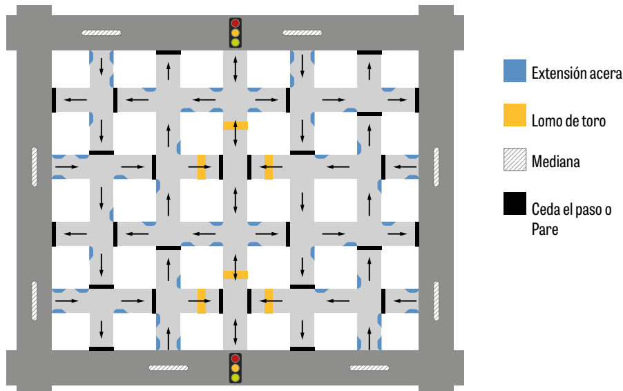
Alternativa 1: modificando el sentido del tránsito y efectuando extensiones de acera
