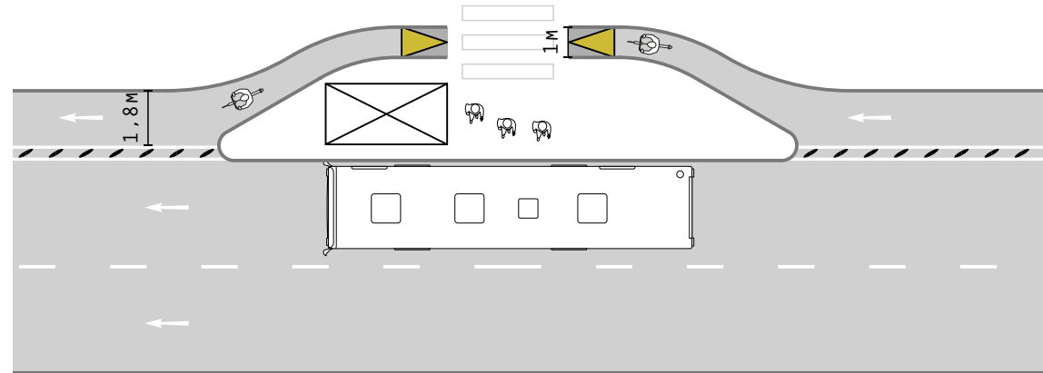
La ciclovía pasa por detrás del paradero, generando una isla para la espera del bus.
