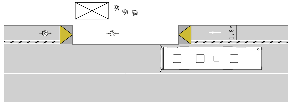
La acera es la zona de espera del bus. Los pasajeros abordan mediante la plataforma, la que actúa al mismo tiempo como zona de calmado de tráfico en la ciclovía.
