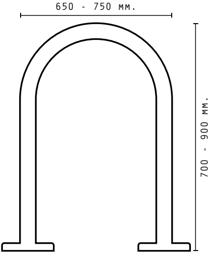
Esquema básico del paradigma de "U Invertida". Para información detallada, remitirse al manual "Biciestacionamientos en el espacio público" (MINVU, 2013).
