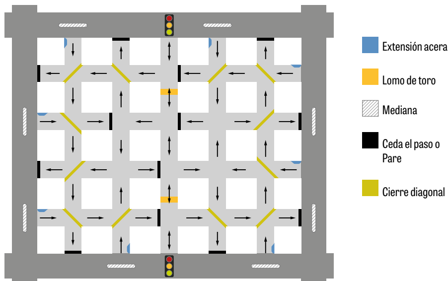
Alternativa 2: modificando el sentido del tránsito y utilizando cierres diagonales con algunas extensiones de acera.
